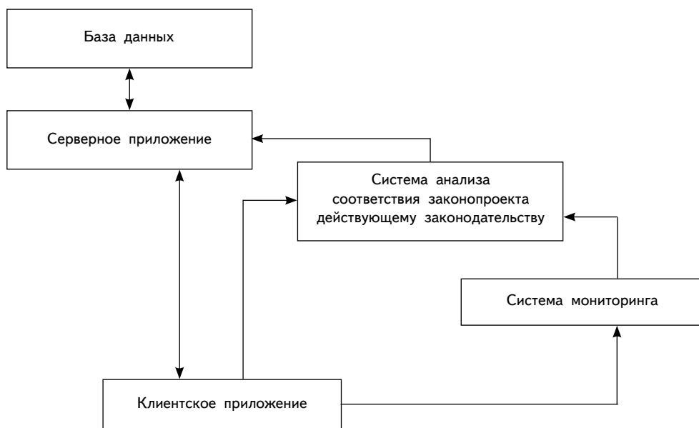
Рис. 1. Структура программного комплекса АИС «Законотворчество» со встроенным модулем «Экспертиза законопроектов»
